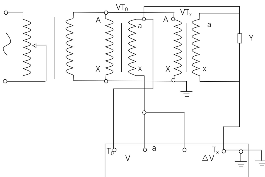
图 2 电压互感器基本误差试验接线
