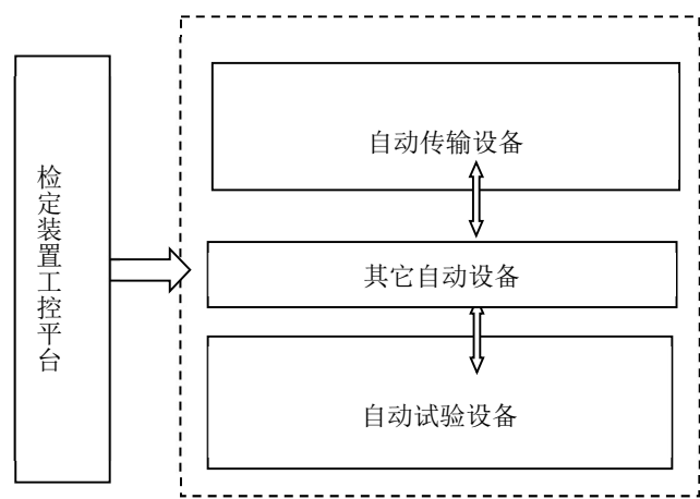
图1 电压互感器自动化检定装置组成示意图
