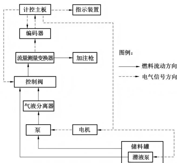
图1 加注机工作原理示意图
